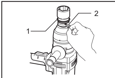
► 1. Anillo-O 2. Clavija
